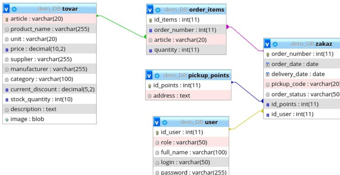
Рисунок 1 – Проект БД
