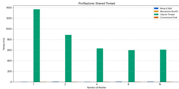
Figure 5. Profilazione con più thread caso Shared
