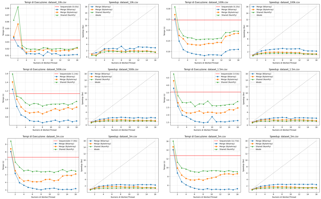
Figure 3. Risultati dei test con dataset di dimensioni crescenti: 10k, 100k, 500k, 1.5M, 3M e 5M email.
