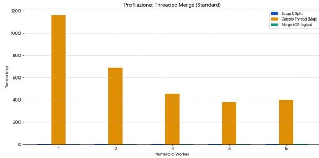
Figure 4. Profilazione con più thread caso standard
