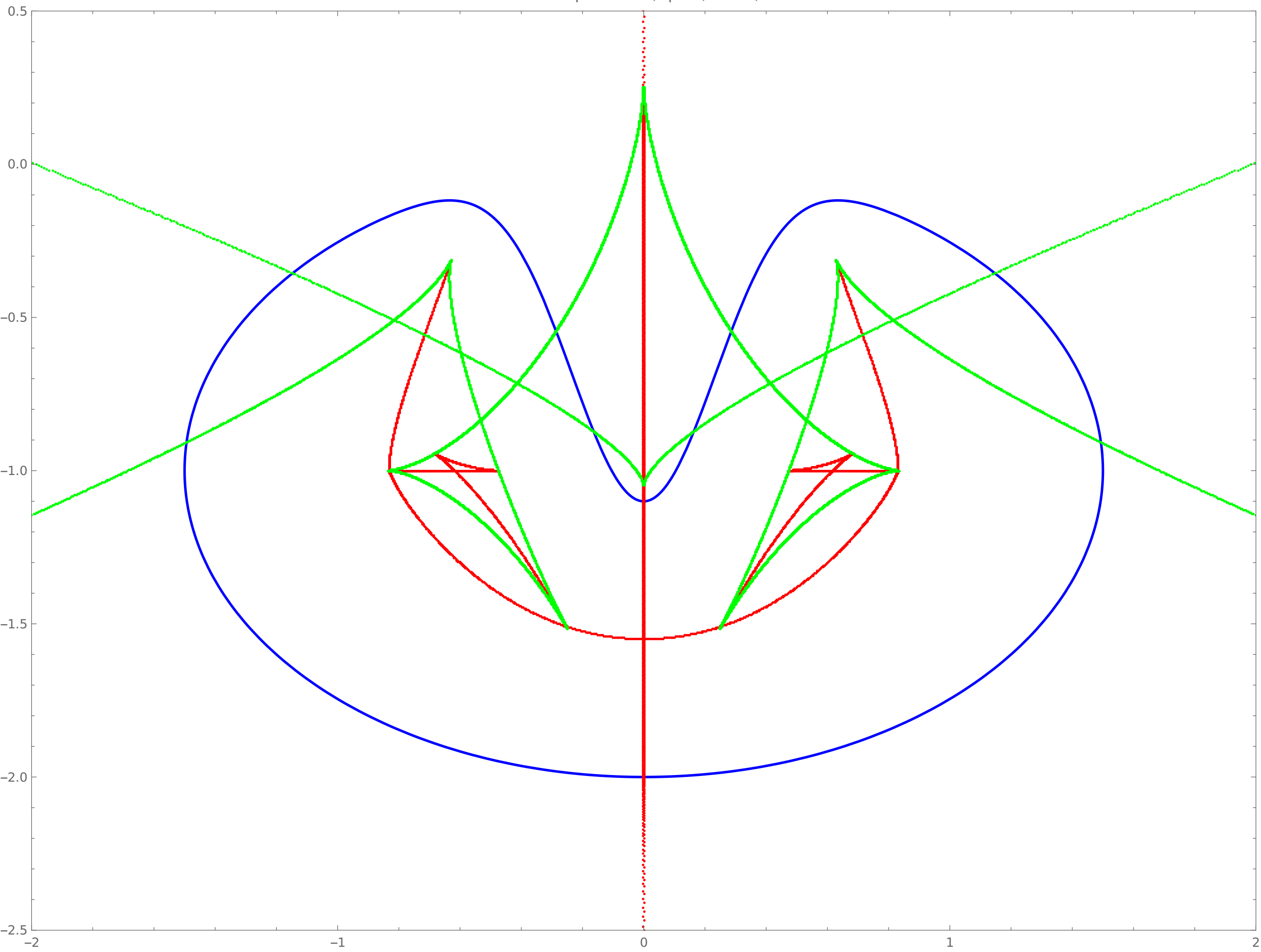
Dented Ellipse H=1 , q=20 , a=1.5 , b=1
