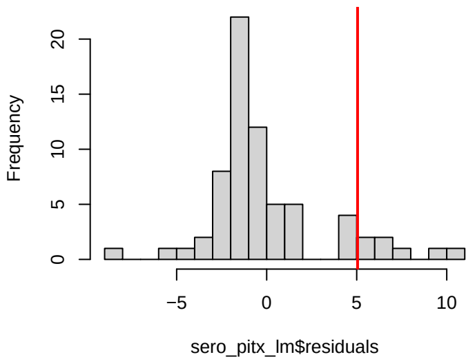
Histogram of sero_pitx_lm$residuals
