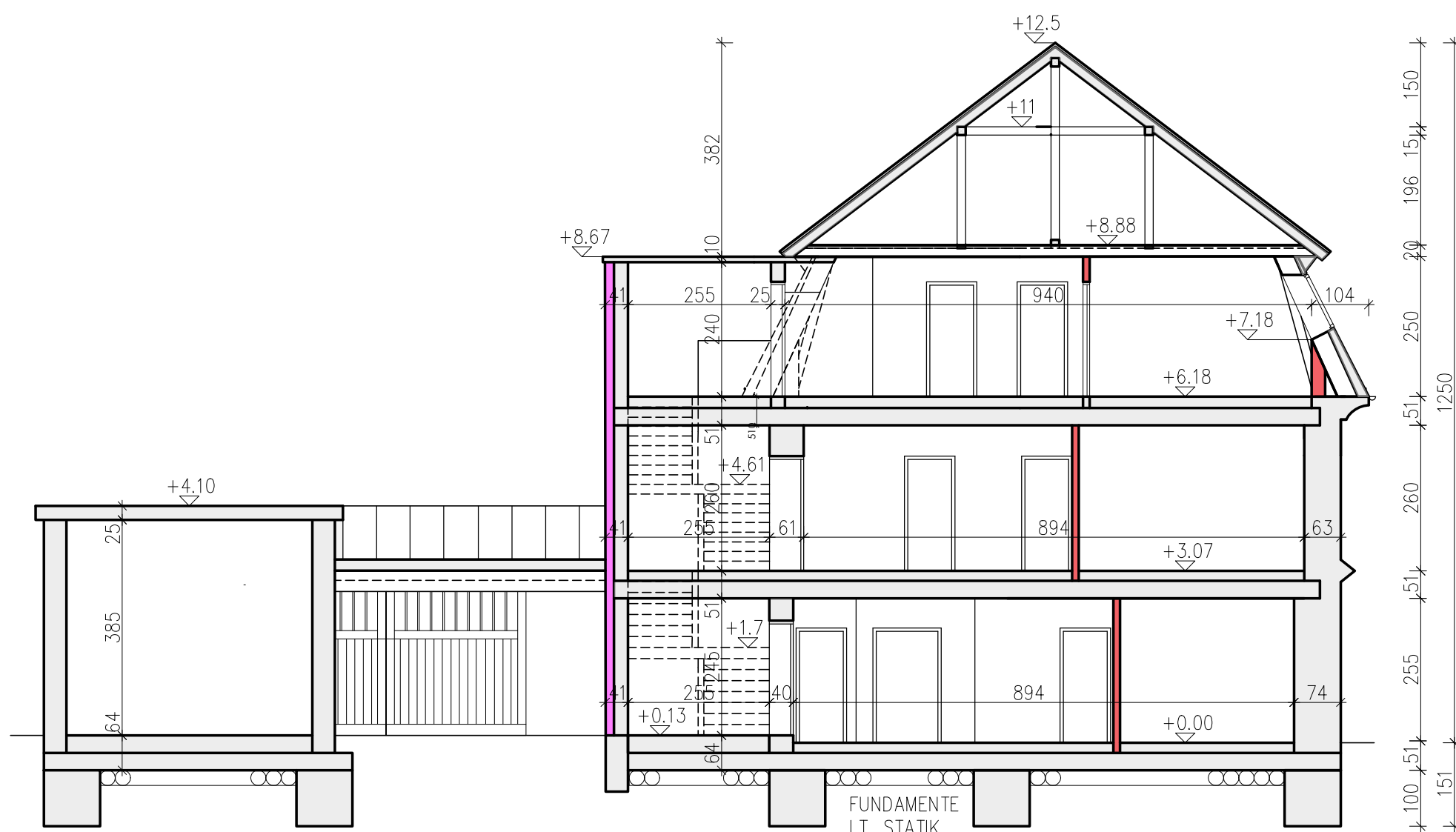
SNITT A-A
