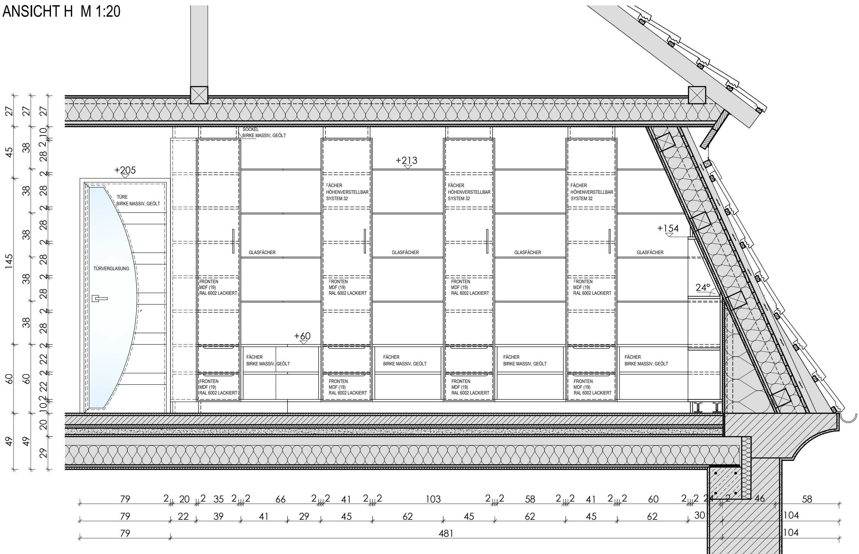
ANSICHT H M 1:20
