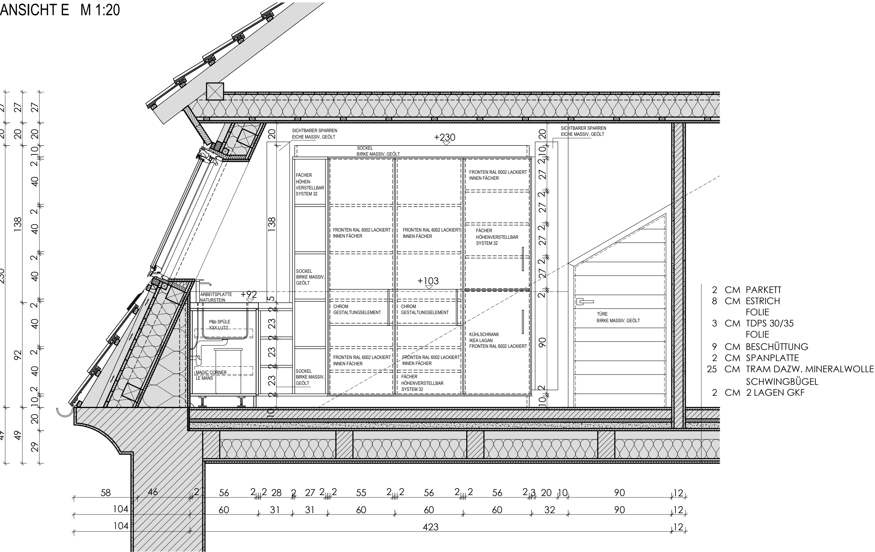
ANSICHT E M 1:20
