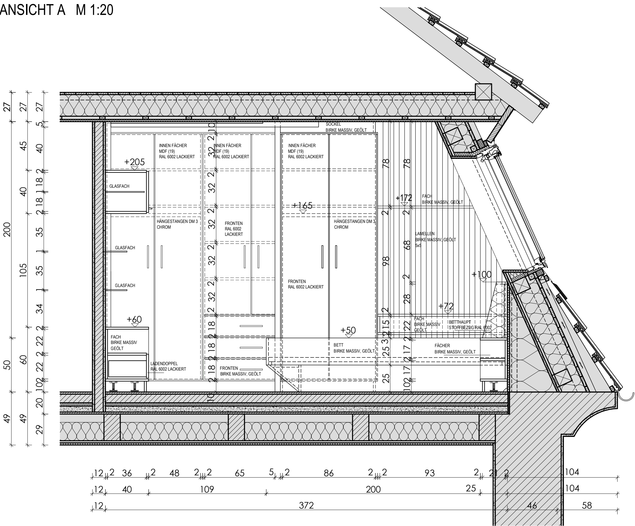
ANSICHT A M 1:20
