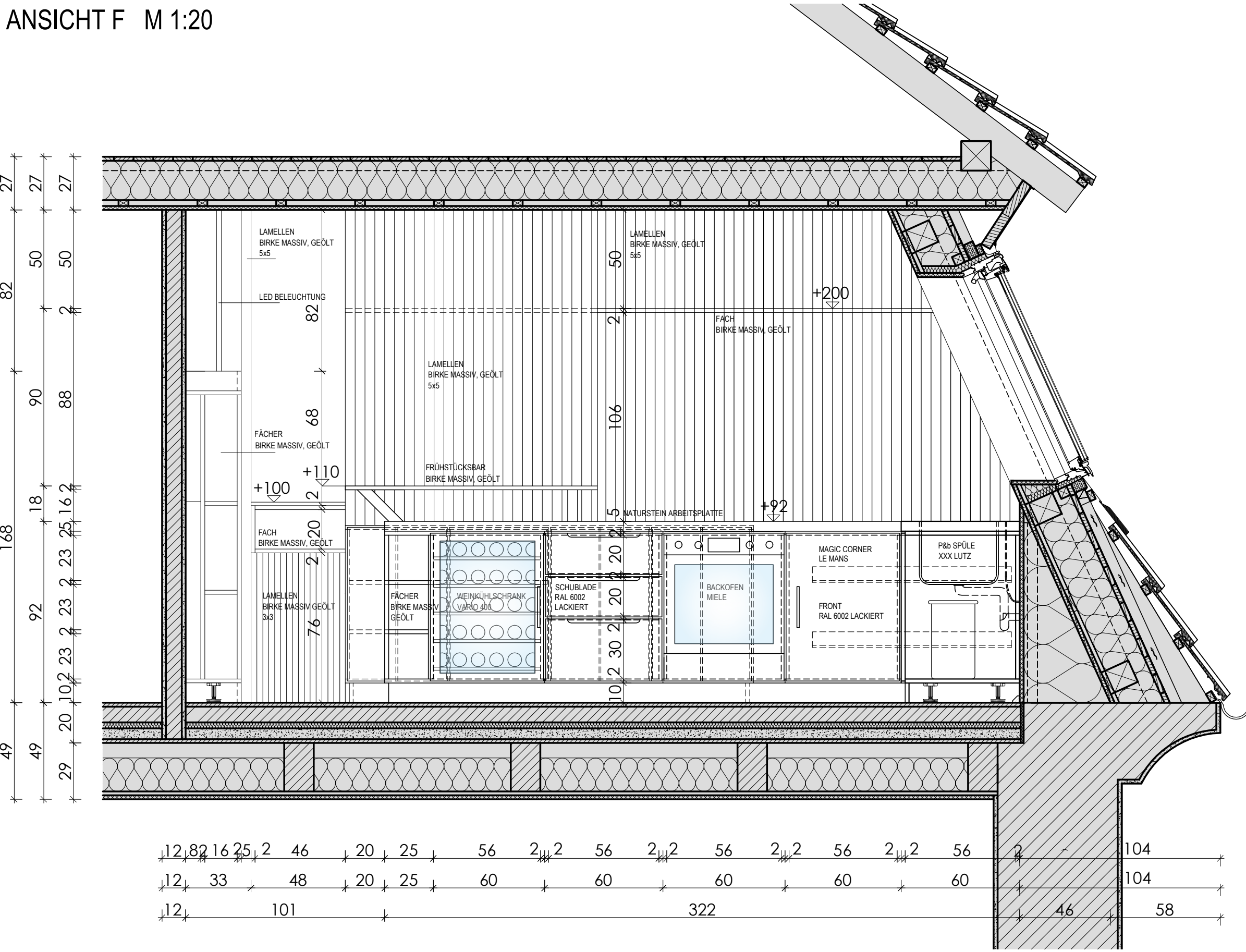
ANSICHT F M 1:20
