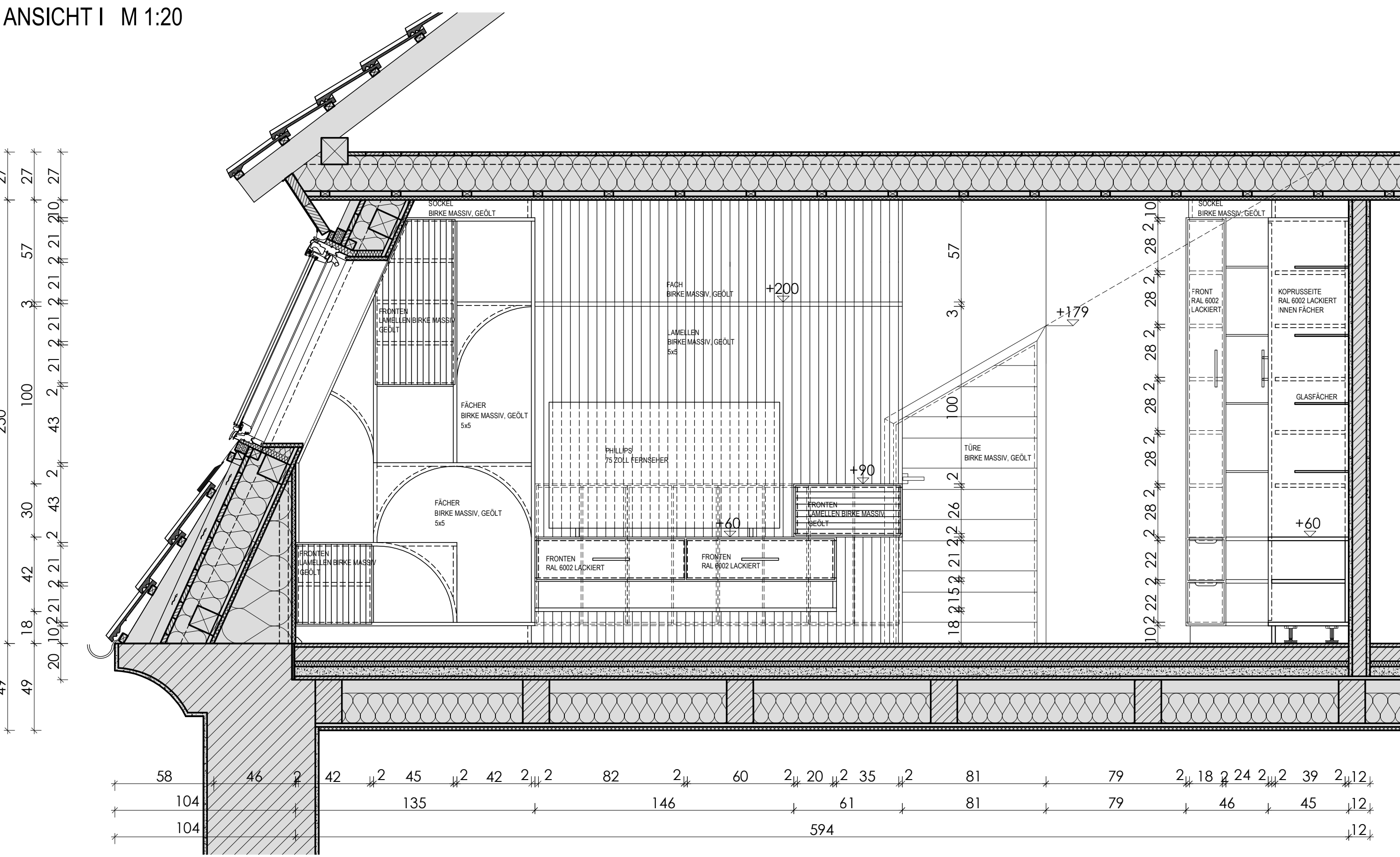
ANSICHT I M 1:20
