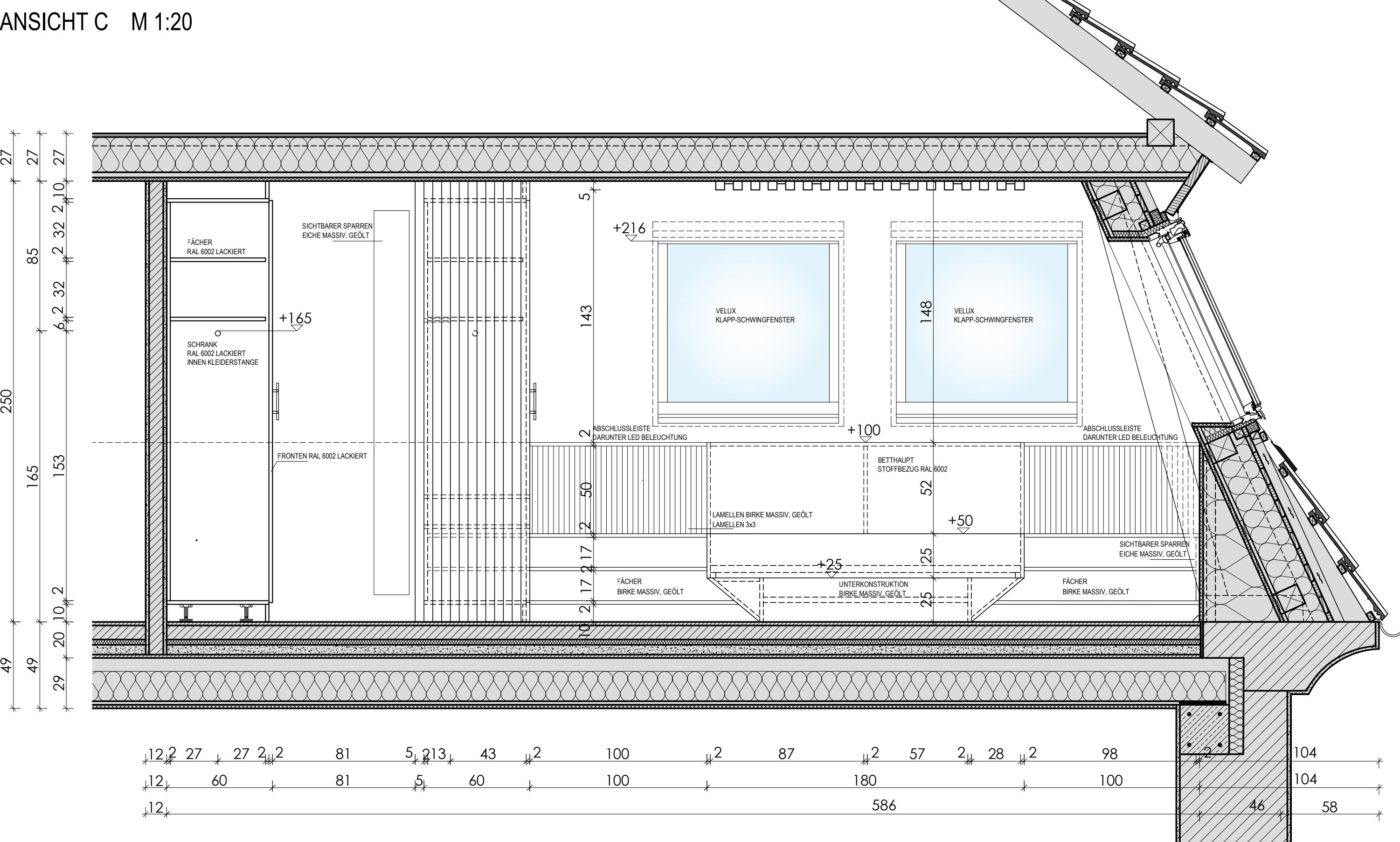
ANSICHT C M 1:20
