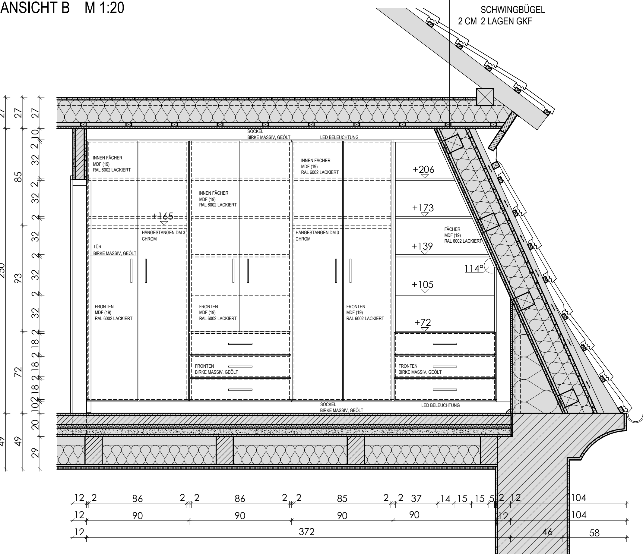
ANSICHT B M 1:20
