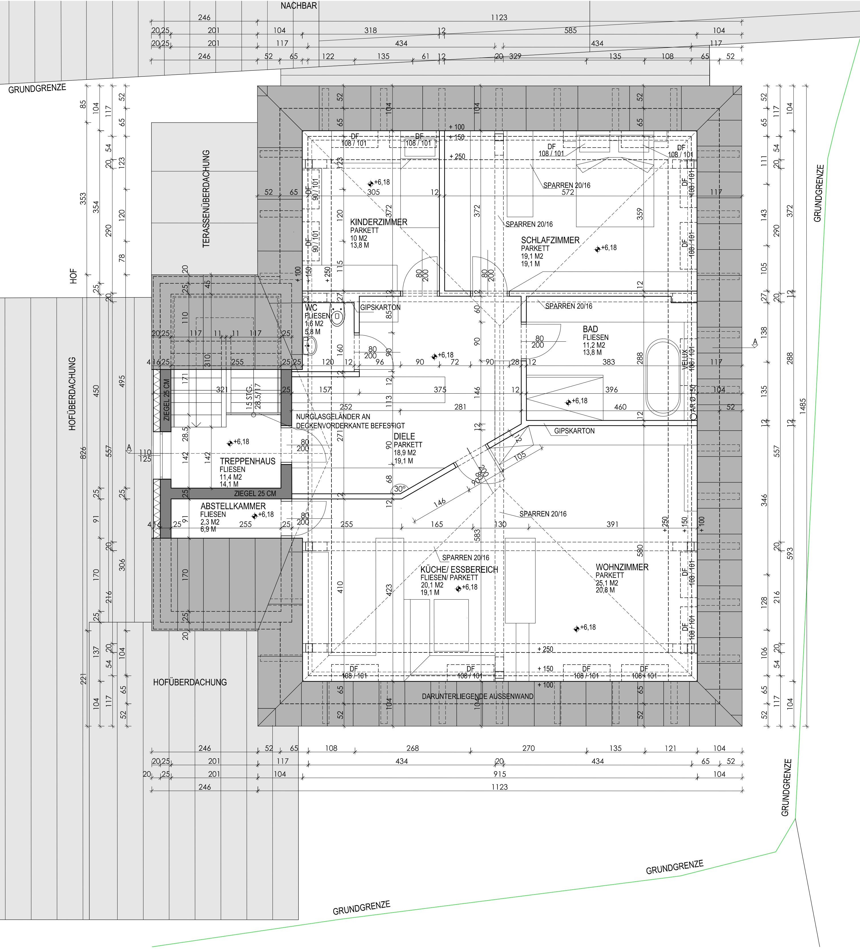
GRUNDRISS DACHGESCHOSS M 1:50
