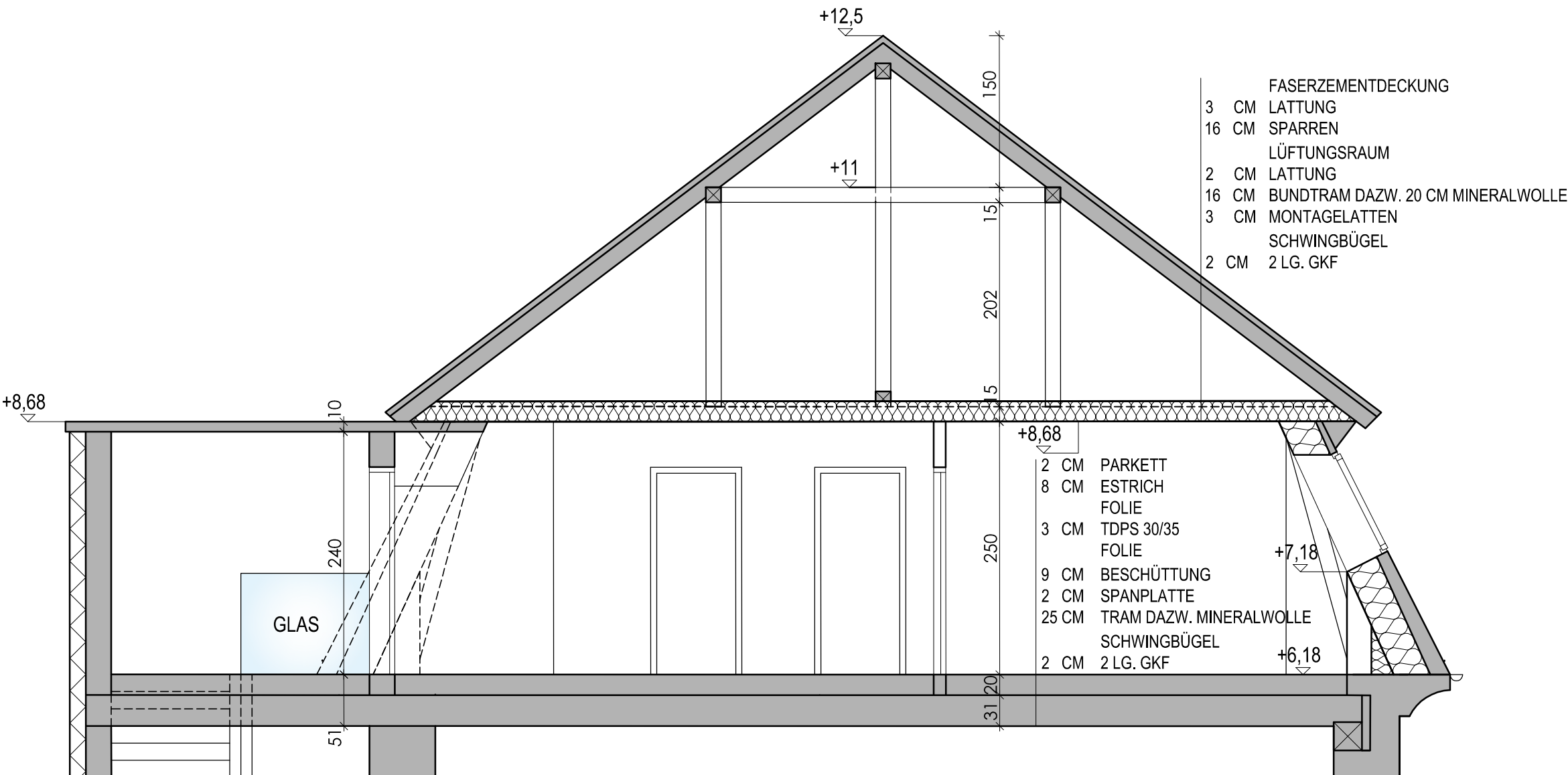
SCHNITT A-A DACHGESCHOSS M 1:50
