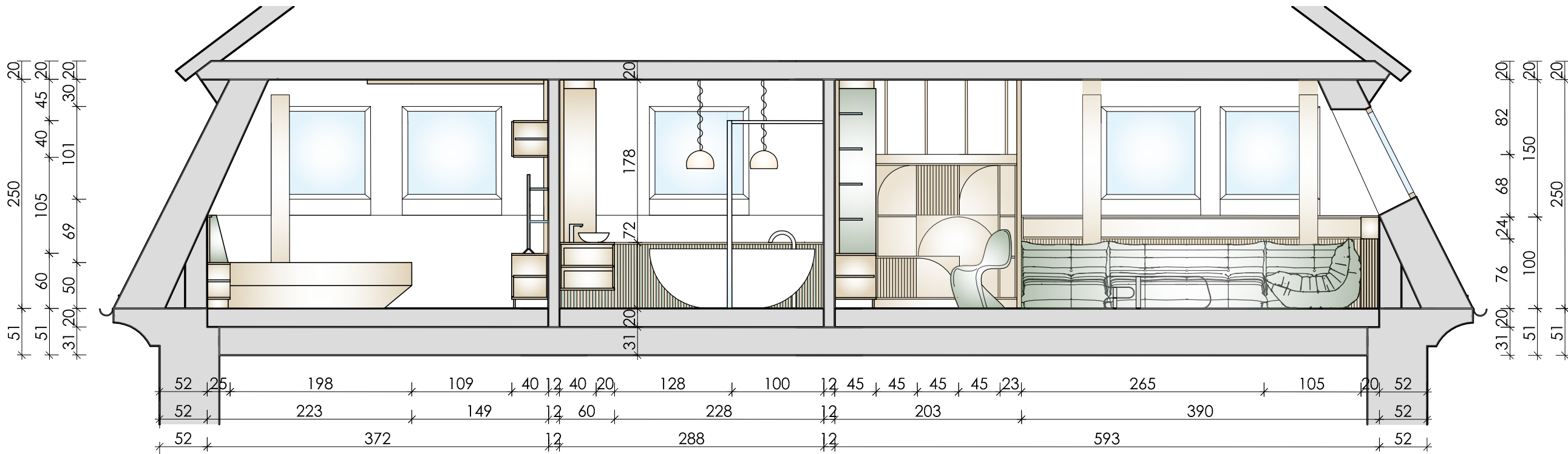
ANSICHT F - F M 1:50
