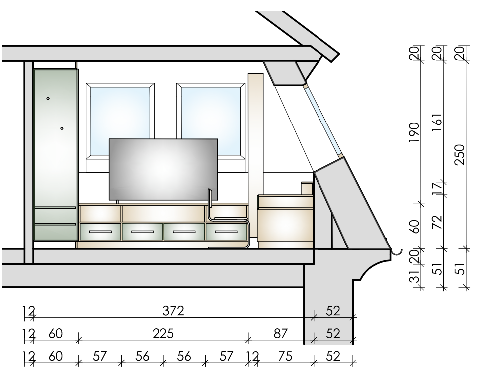
ANSICHT I - I M 1:50
