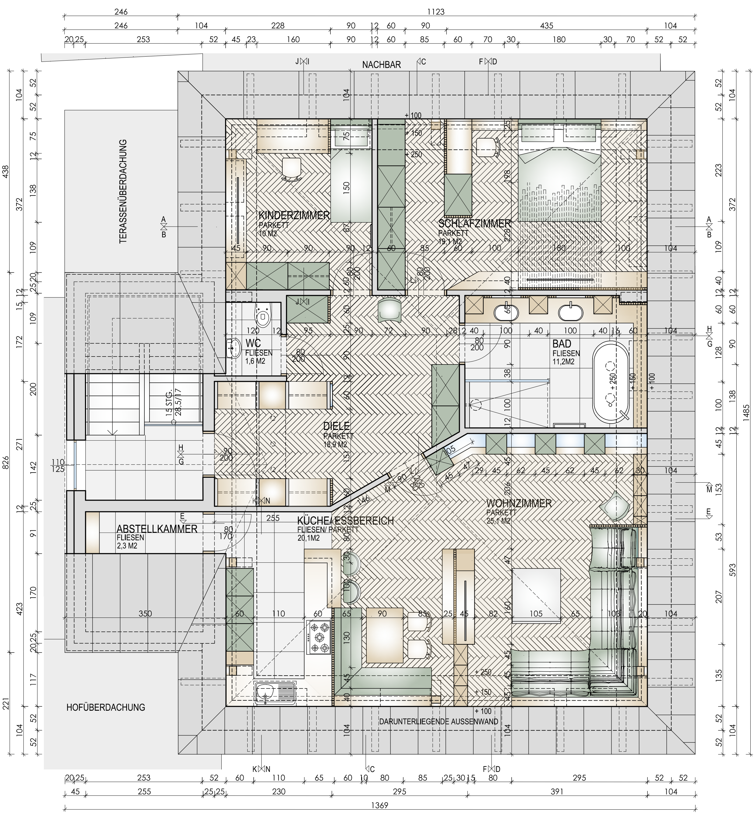
GRUNDRISS DACHGESCHOSS M 1:50
