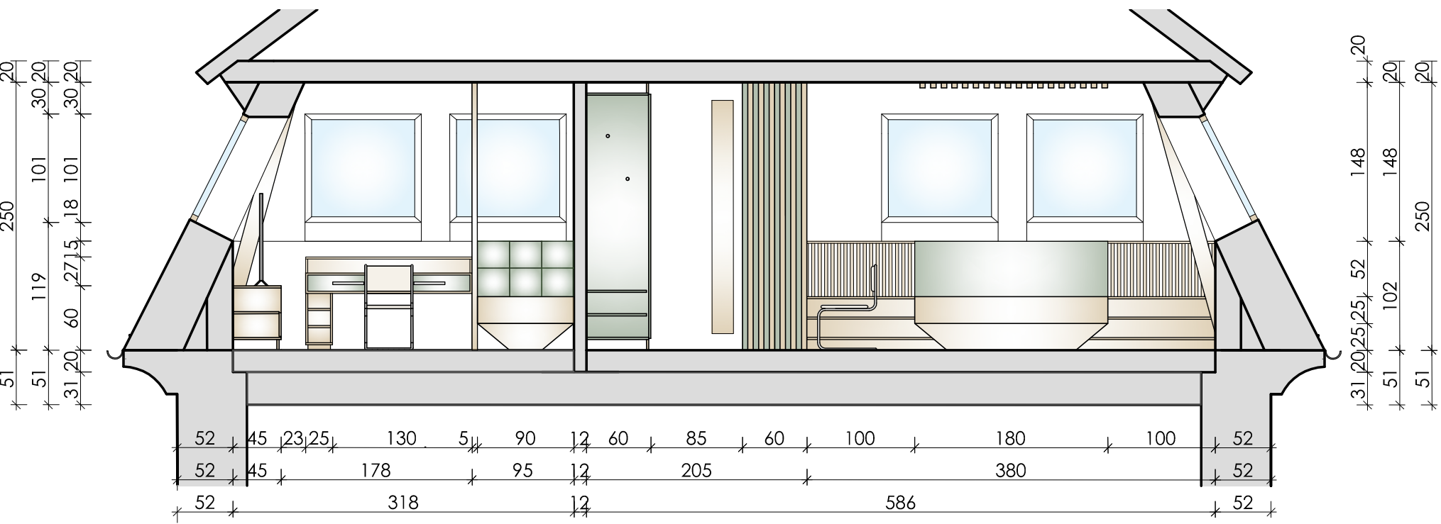
ANSICHT A - A M 1:50
