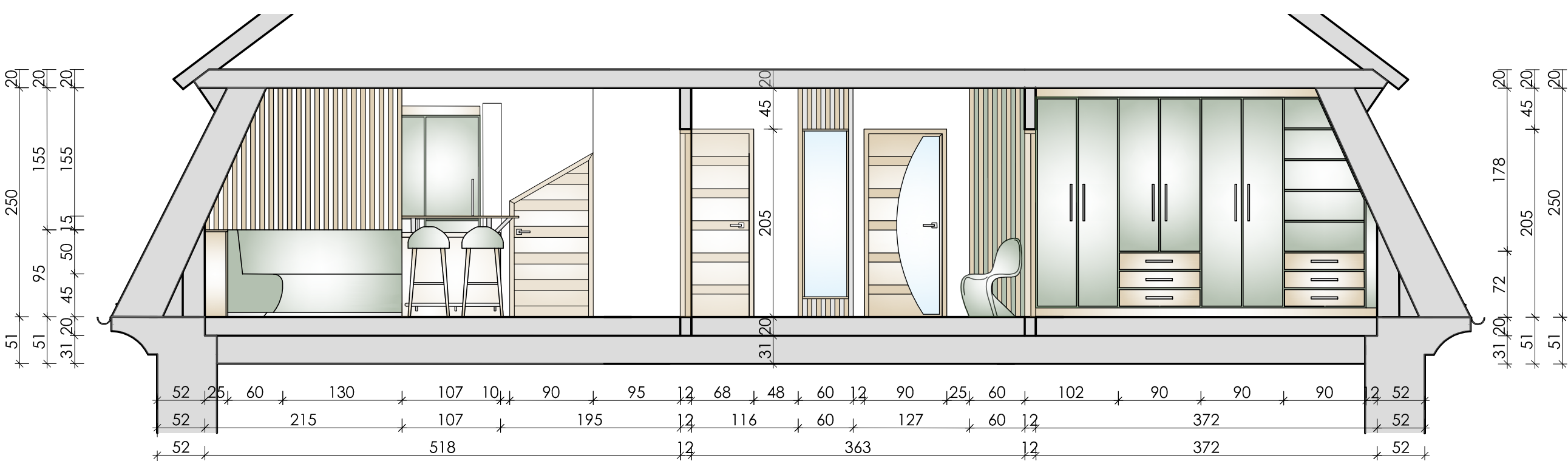
ANSICHT C - C M 1:50
