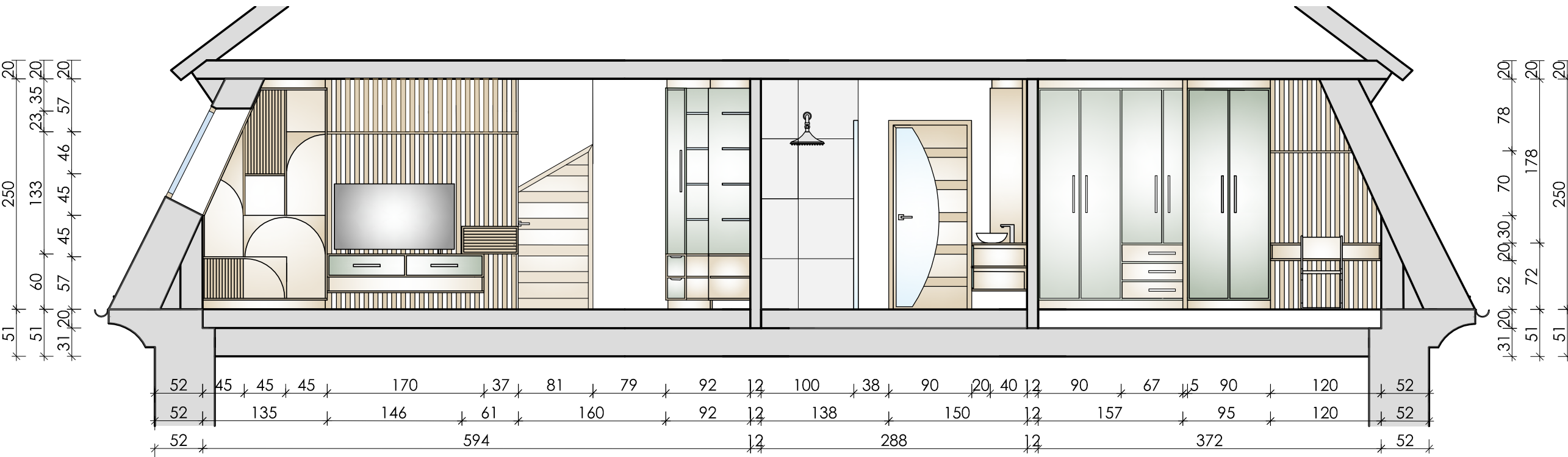
ANSICHT D - D M 1:50
