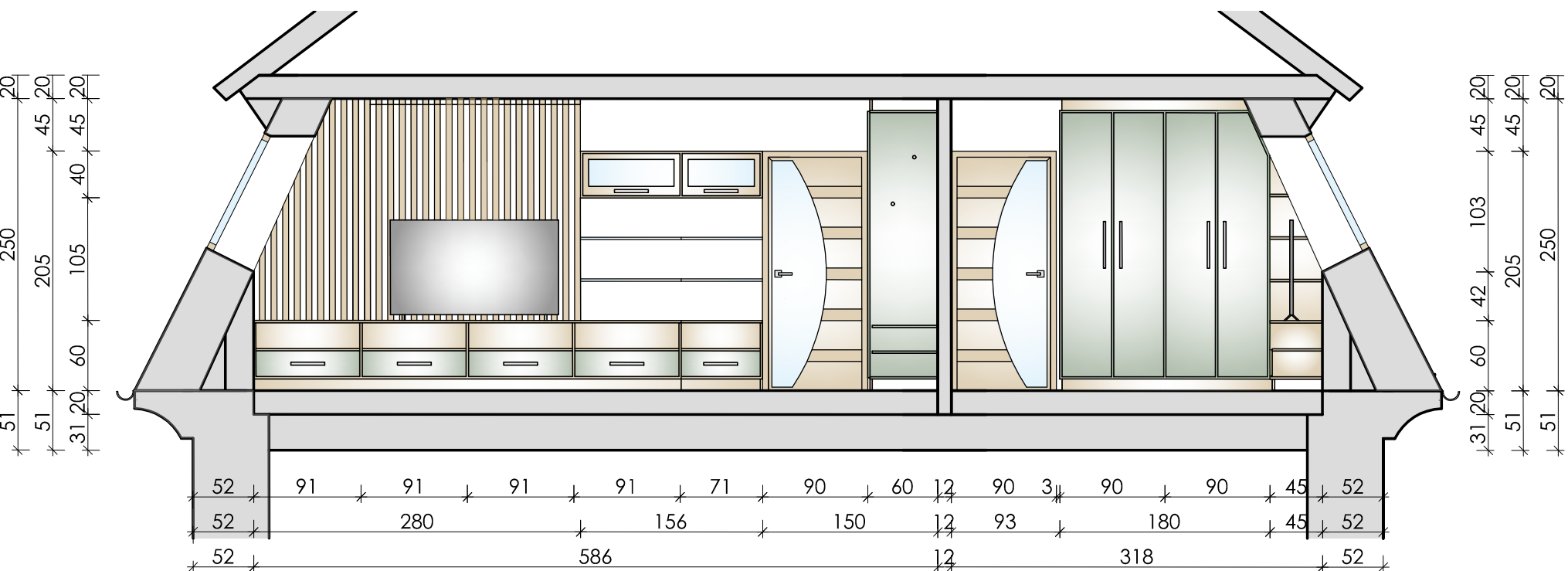
ANSICHT B - B M 1:50
