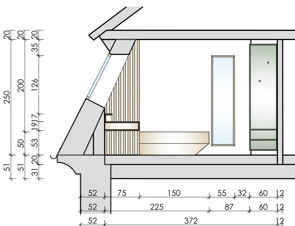
ANSICHT J - J M 1:50
