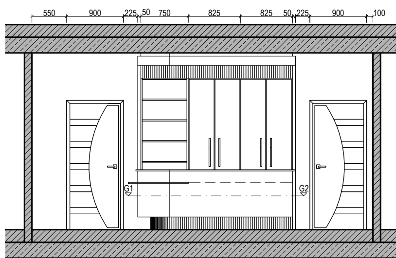
ANSICHT B M 1:50
