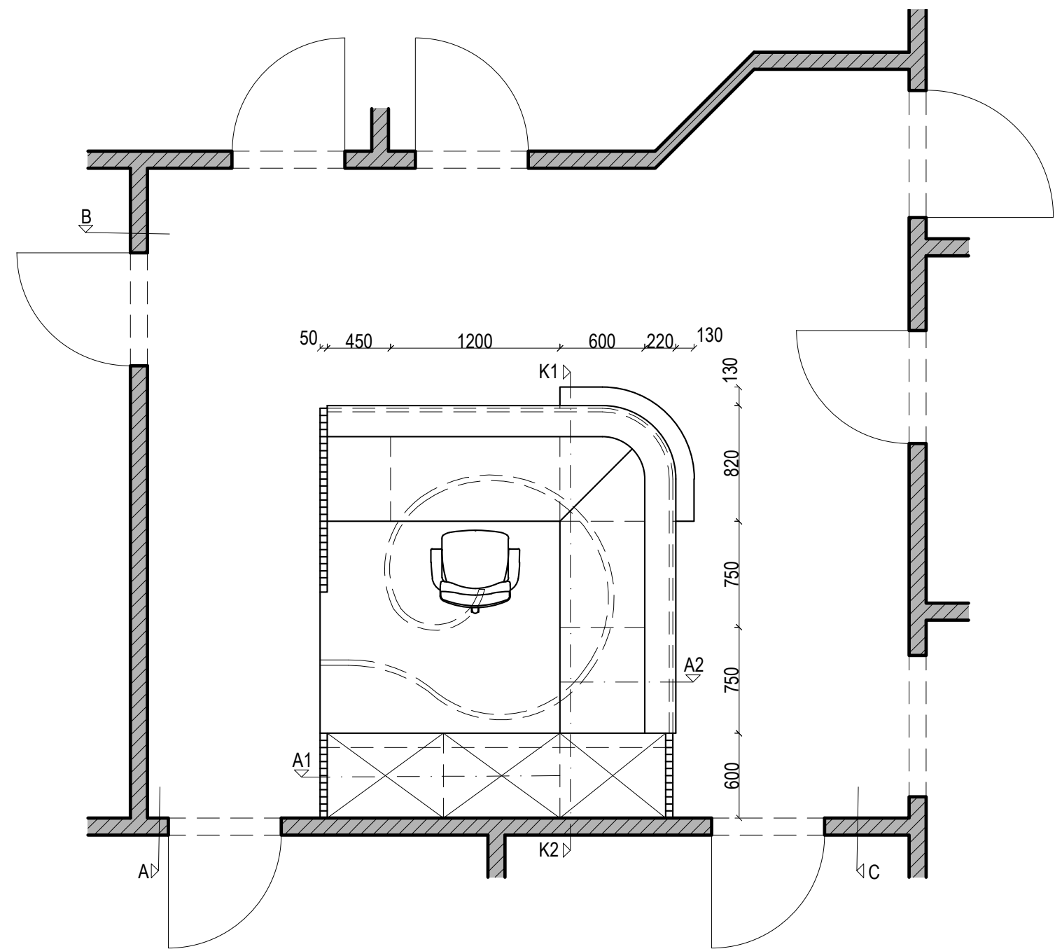
ÜBERSICHT GRUNDRISS M 1:50
