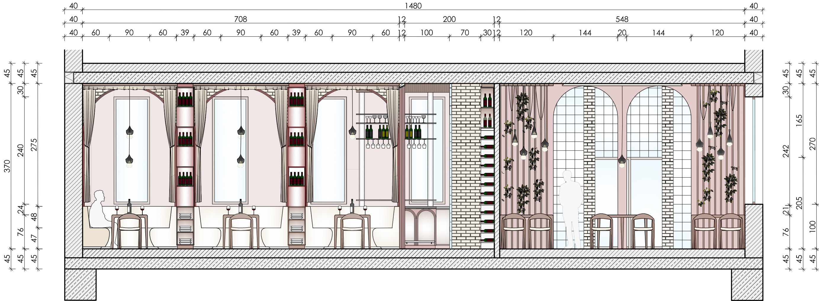
ANSICHT A-A M1:50
