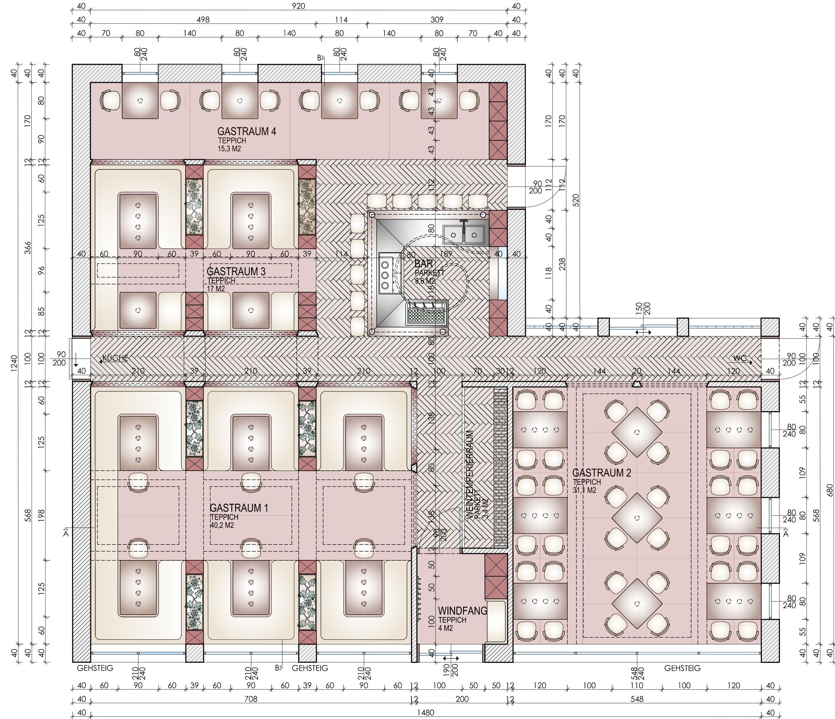
GRUNDRISS M1:50
