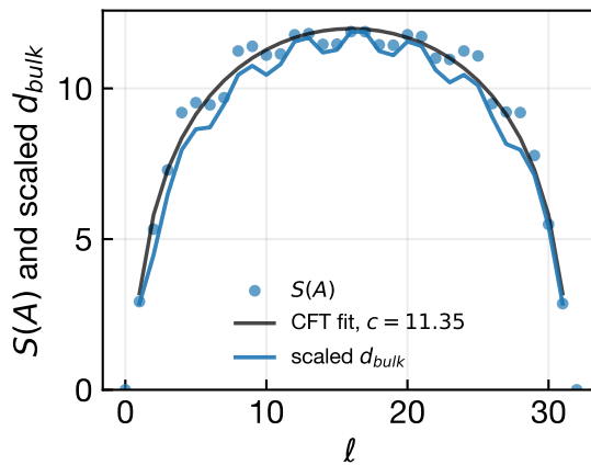
(d) \mu = 0.1
