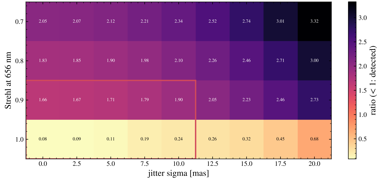
detectable flux / F(PDS 70 b), 180 mas, 1 h, 2 nm
