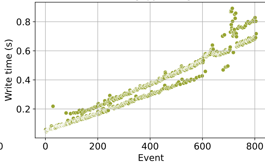
iceberg (pyiceberg)
