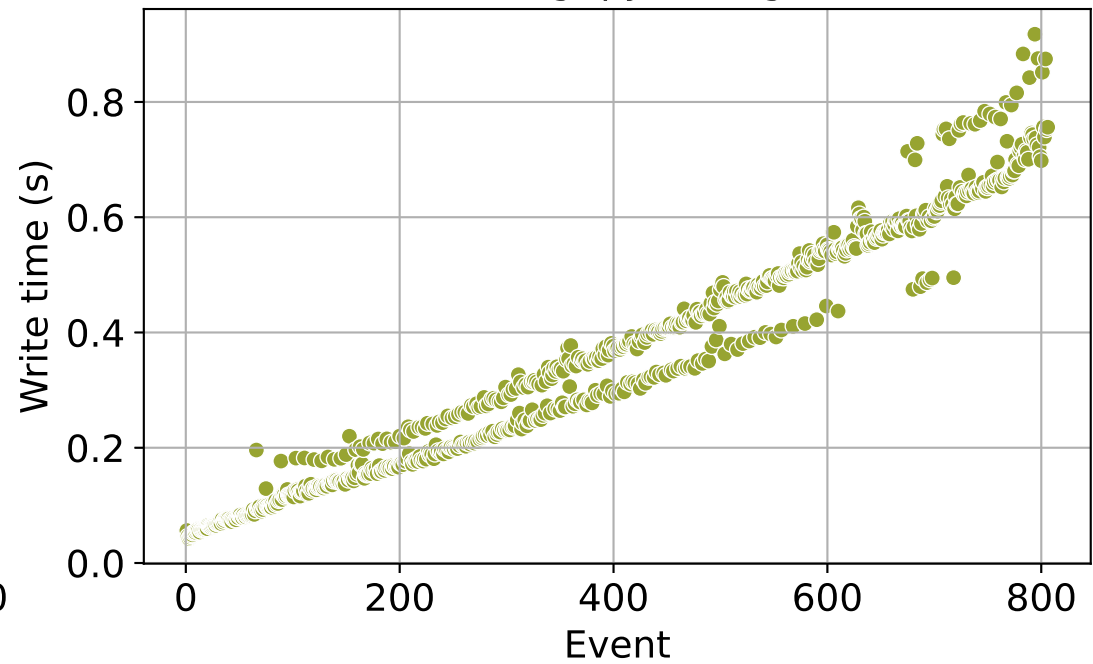
iceberg (pyiceberg)
