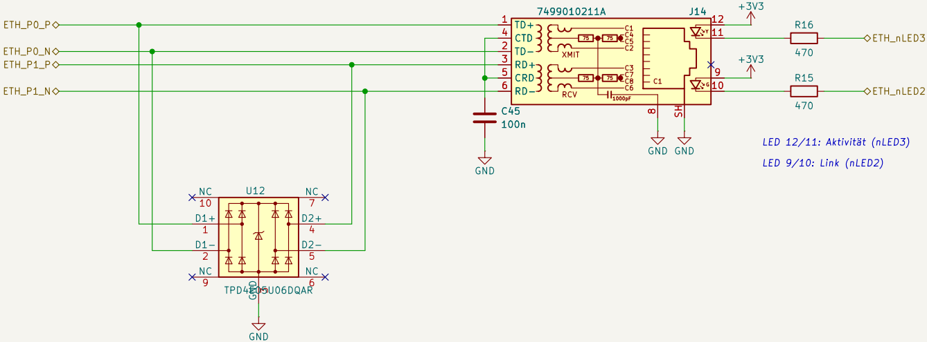
MagJack 1:1 wie CM4–Datenblatt (Figure 2): Mittelanzapfungen über C45 an GND, ESD–Schutz U12, LED 470 Ω 10/100 genügt für VoIP; für Gigabit 4–Paar–MagJack verwenden und Paare 2/3 des CM4 anschließen
