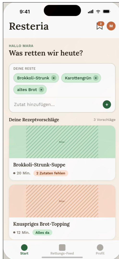
Abb. 1. UI/UX-Mockup Resteria: Startseite mit Reste-Eingabe und Rezeptvorschlag
