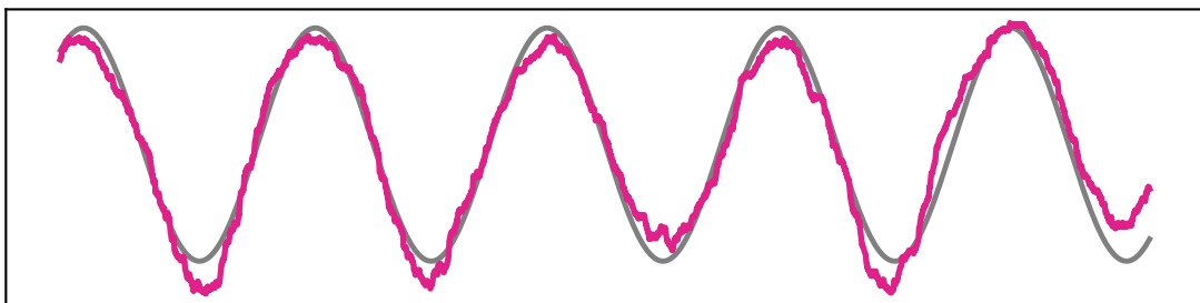
Time (samples)
