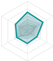
6. drsr (30.4)
