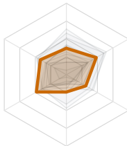
8. gplearn (25.8)
