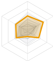
7. llmsr (30.0)
