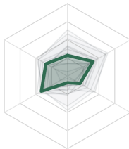
12. ragsr (11.1)
