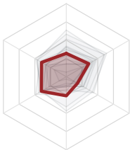
9. pyoperon (23.4)
