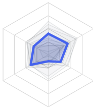
11. e2esr (20.4)
