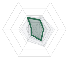
12. ragsr (11.1)
