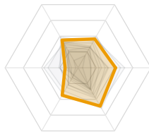
7. llmsr (30.0)
