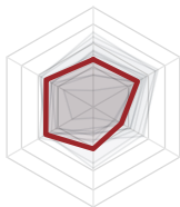
9. pyoperon (23.4)
