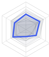
11. e2esr (20.4)
