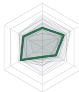
12. ragsr (11.1)
