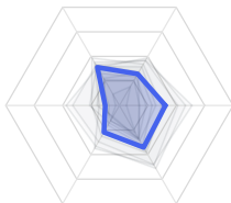
11. e2esr (20.4)
