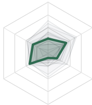
12. ragsr (11.1)
