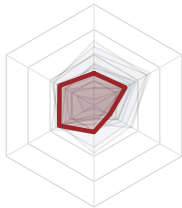
9. pyoperon (23.4)
