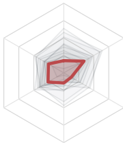
11. e2esr (20.4)
