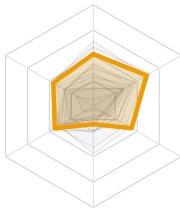
7. llmsr (30.0)
