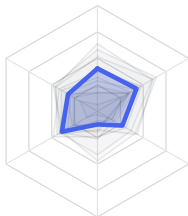
11. e2esr (20.4)
