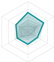
6. drsr (30.4)
