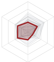
9. pyoperon (23.4)
