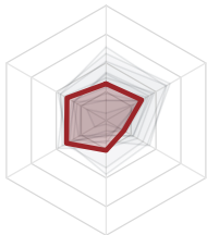
9. pyoperon (23.4)
