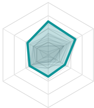
6. drsr (30.4)
