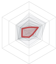
11. e2esr (20.4)
