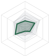
12. ragsr (11.1)
