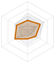
8. gplearn (25.8)
