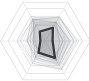
12. ragsr (11.1)
