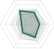
12. ragsr (11.1)
