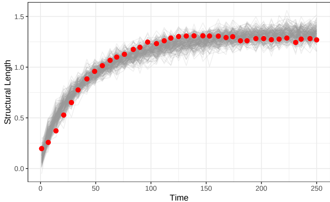
Posterior Predictive Check: Growth
