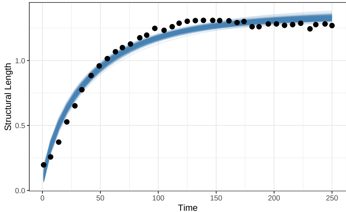
Posterior Predicted Trajectories
