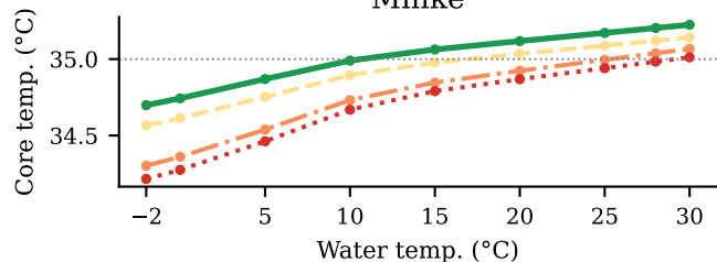
Minke
