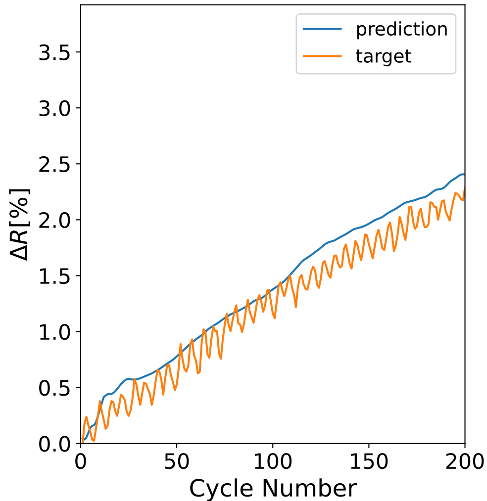
Sense A: MAE=0.16, R2=0.91
