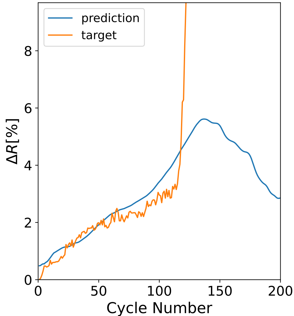
Sense A: MAE=0.42, R2=0.73
