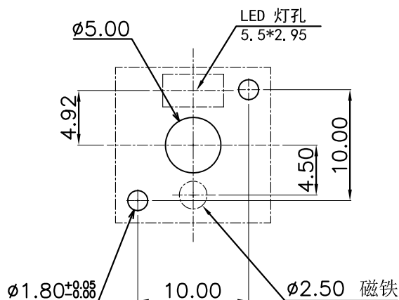
PCB开孔图(供参考)
