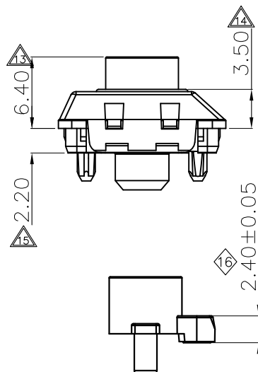
导芯组装磁铁高度尺寸
