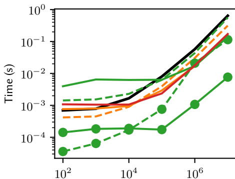
scipy.signal.welch
