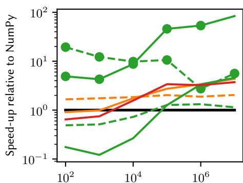
scipy.signal.welch
