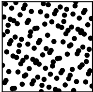
C) Halton
