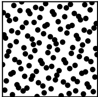
B) Sobol'
