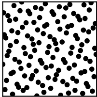
B) Sobol'
