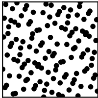
C) Halton
