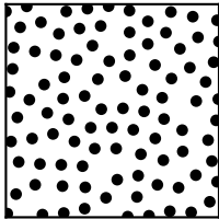
D) Latin hypercube
