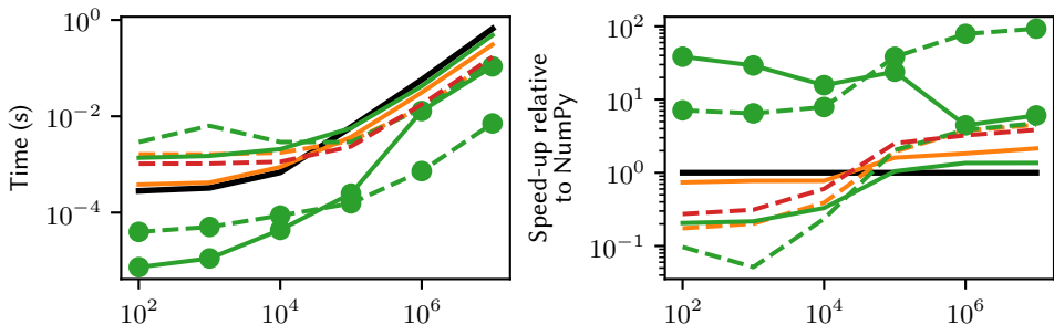
b) scipy.signal.welch
