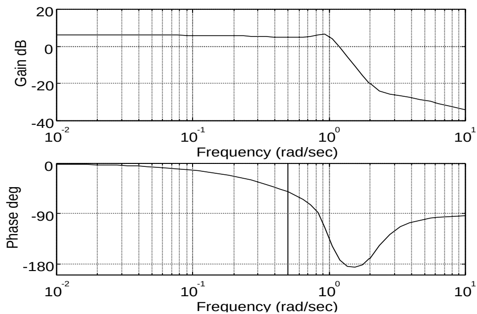
Figura 3. Ejemplo de diagrama de bode de lazo abierto del sistema de regulación de velocidad
