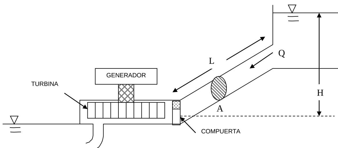
Figura 1. Esquema de una planta hidráulica
