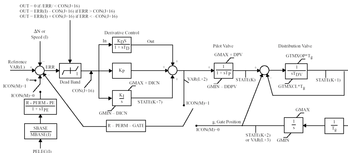
Figura 4. Ejemplo de diagrama de bloques del regulador de velocidad PID y turbina
