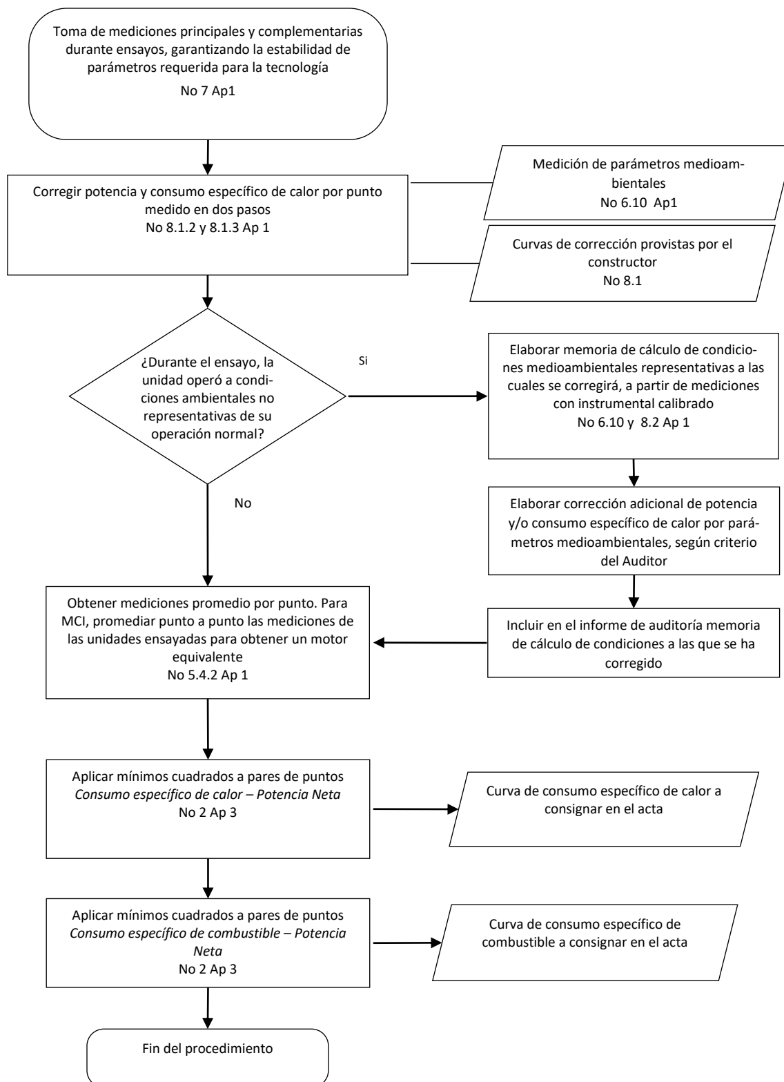
Diagrama de flujo del procesamiento de las mediciones
