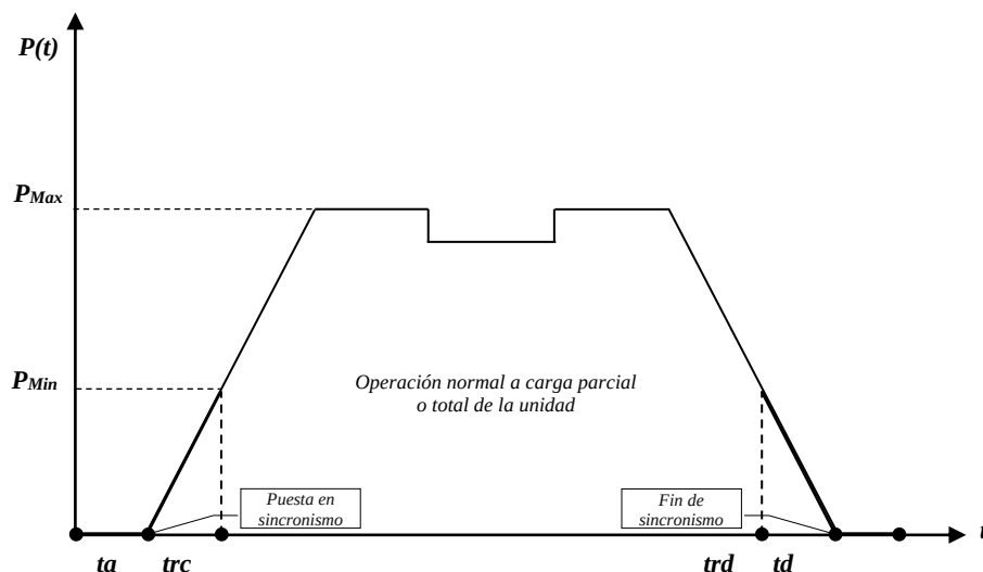
Figura 1 - Ciclo de arranque y detención
