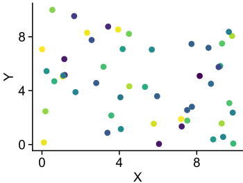
mpl_scatter
