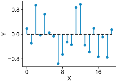
mpl_stem
