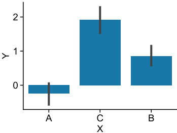
sns_barplot
