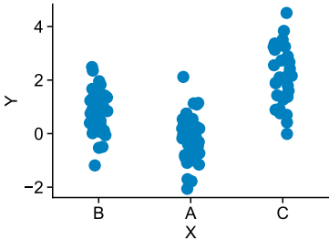
sns_striplot
