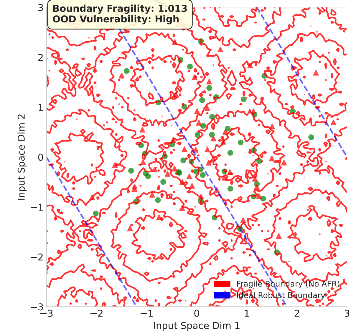
(d) Missing AFR: Fragile Decision Boundaries
