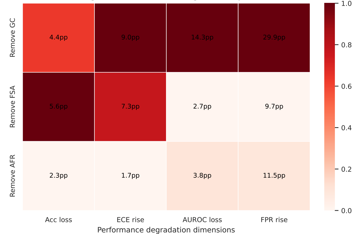
(d) Degradation After Removing One Component
