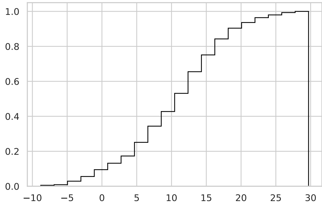
ECDF
