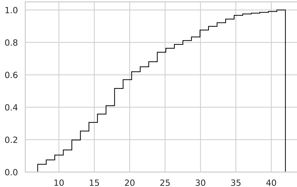
ECDF
