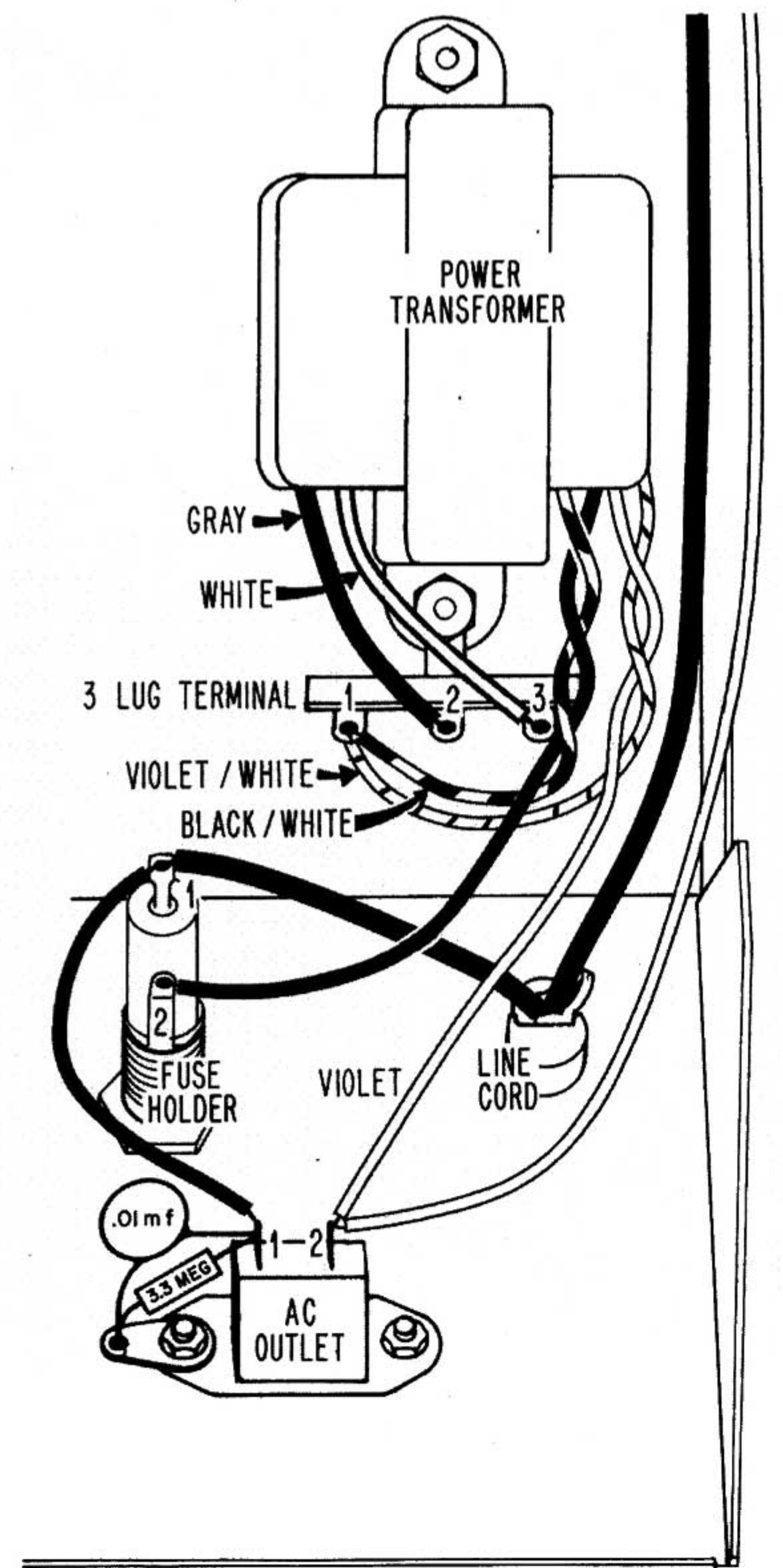
240 VOLT AC WIRING
