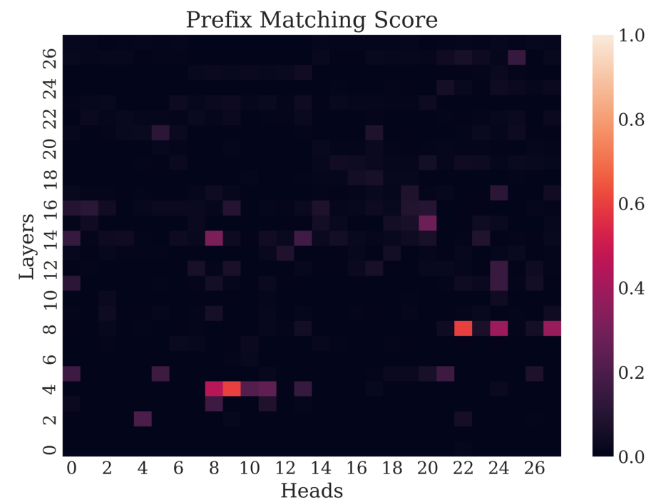
(h) Qwen2.5-VL-7B-Instruct (img tokens) 0.600
