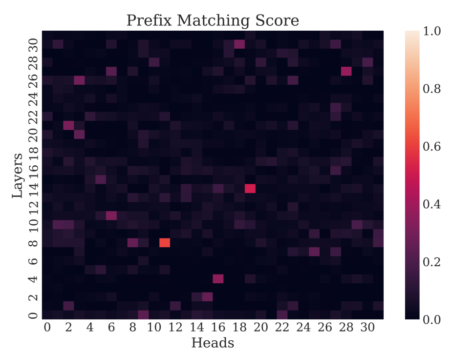
(d) Llama-3.2-11B-Vision-Instruct (img tokens) 0.612
