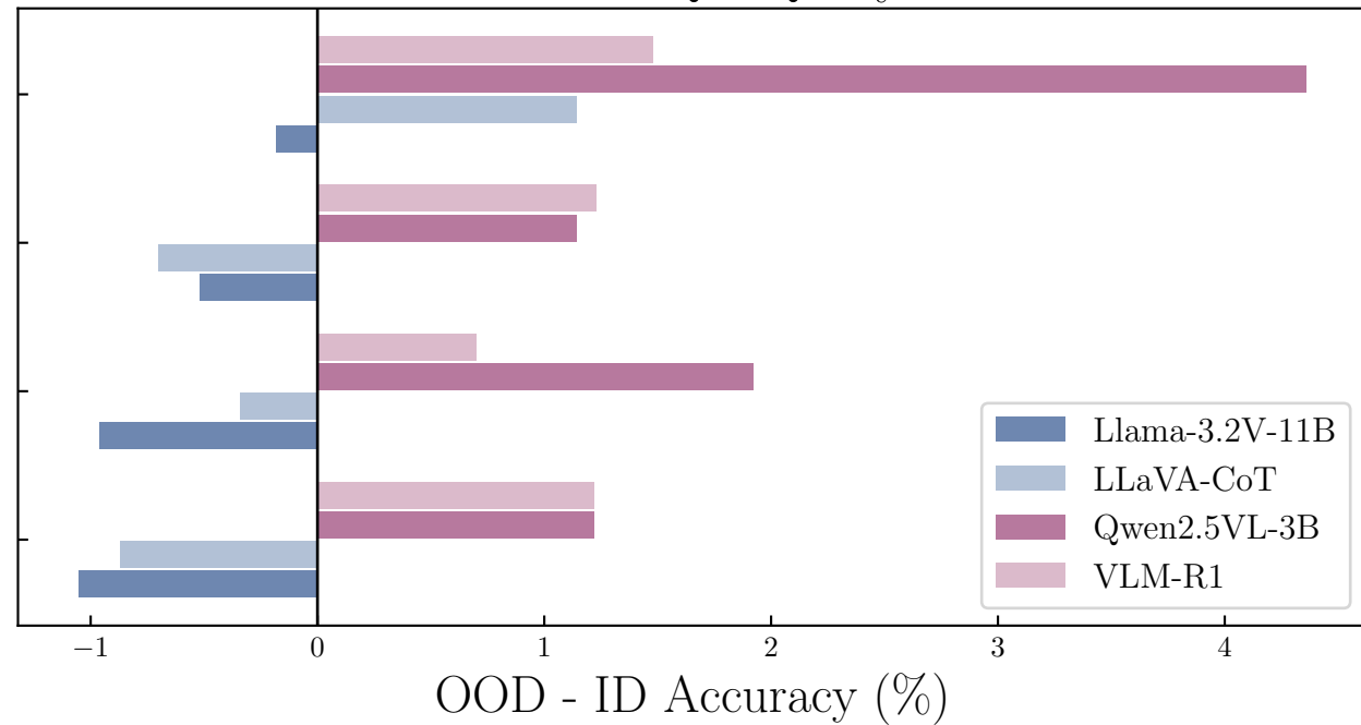
A-OKVQA Query
