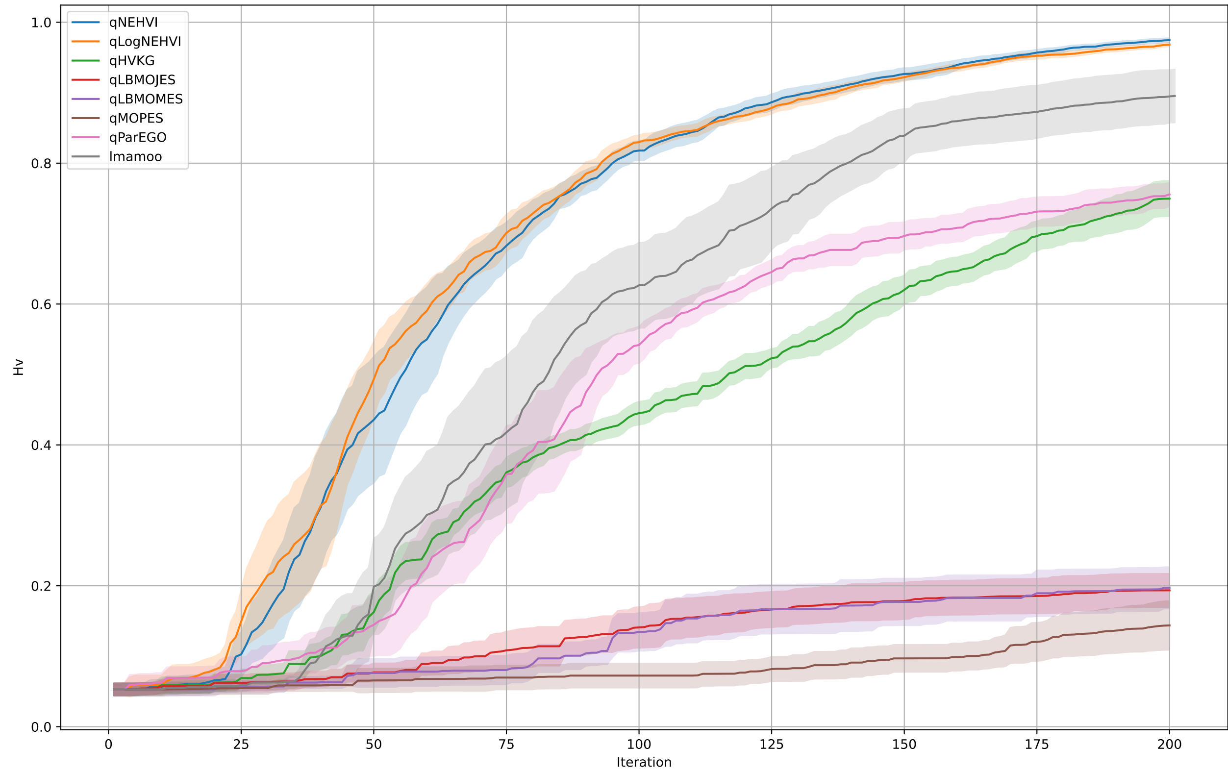
DTLZ2
