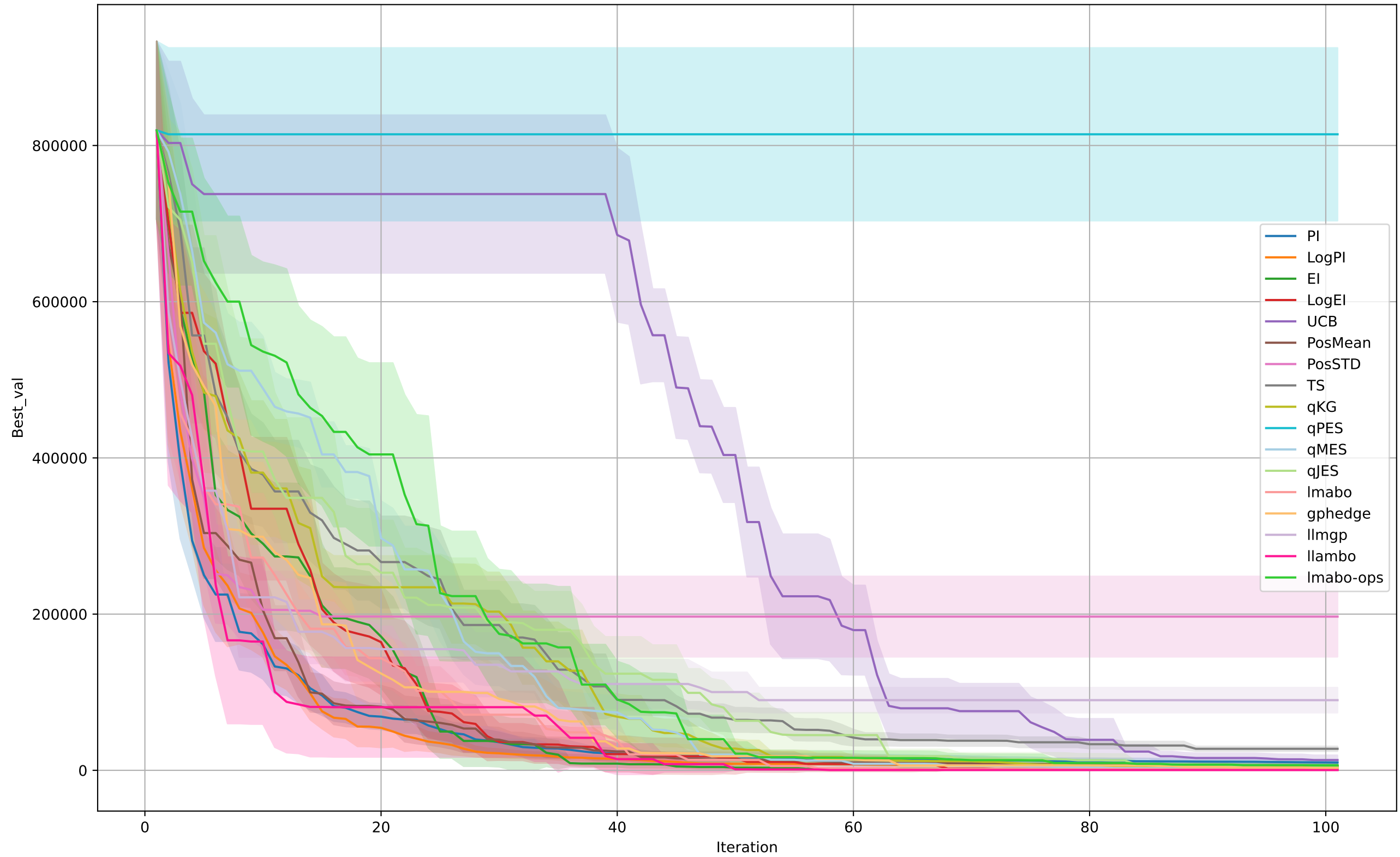
DixonPrice
