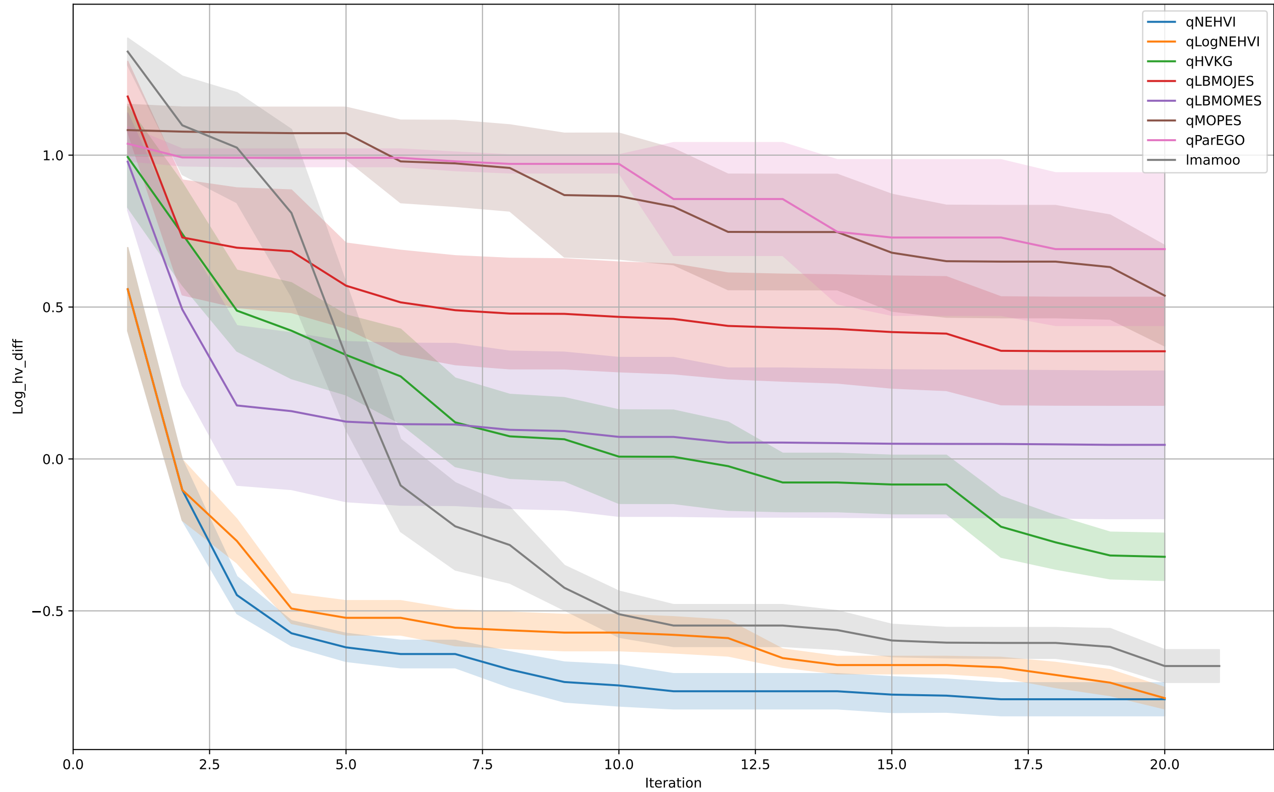
ZDT1
