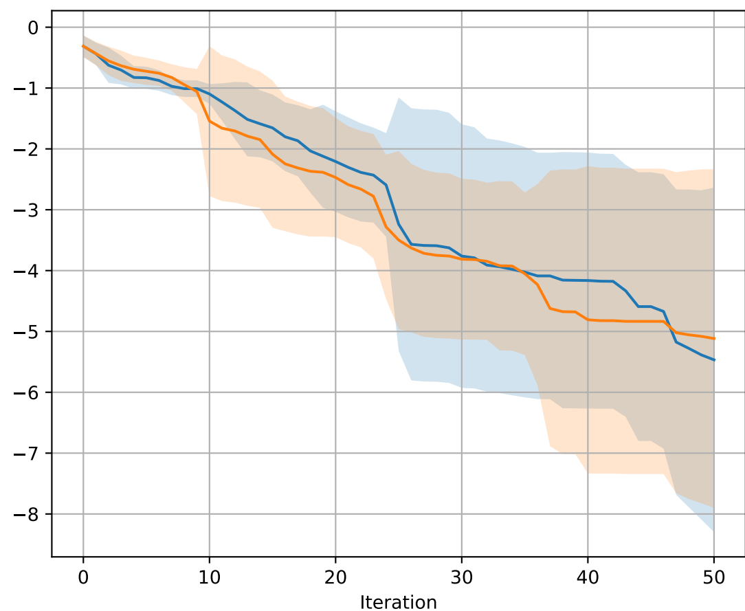
hpt_diabetes_DecisionTree
