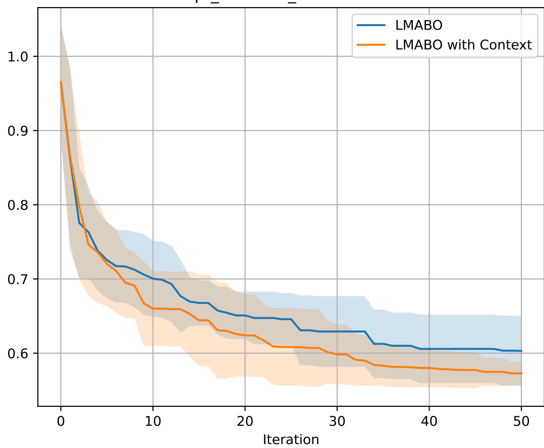
hpt_diabetes_DecisionTree
