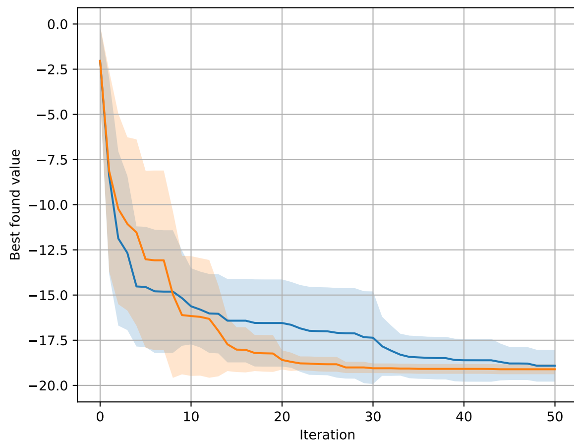
hpt_digits_DecisionTree
