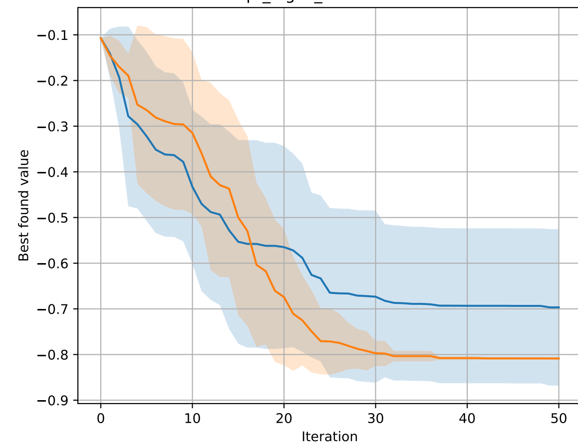
hpt_digits_DecisionTree
