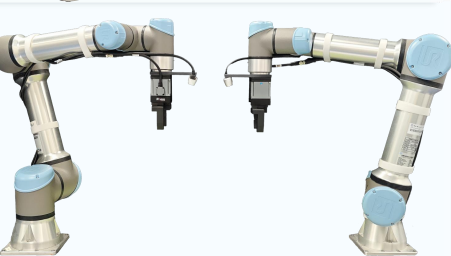
Dual UR5e-Gripper
